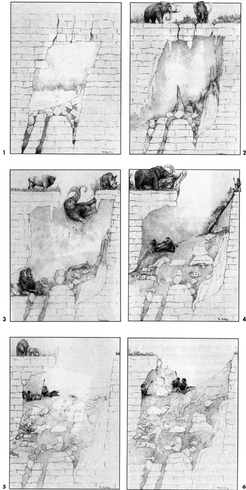
Fig. 2: Évolution du système karstique de Romain-la-Roche et genèse du site, d'après un dessin de T. BALLAY publié par P. PAUPE (1995) puis T. MALVESY (2008).
